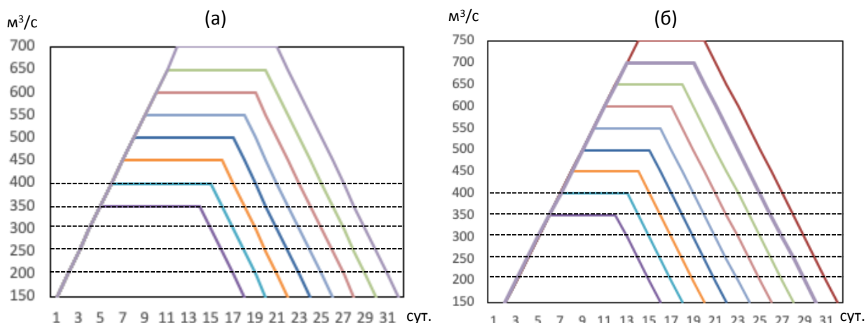
Рисунок 5. Гидрографы попусков различного объема с десятидневной (а) и семидневной (б) продолжительностью пика и суточным изменением расхода на подъеме и спаде 50 м³/с
