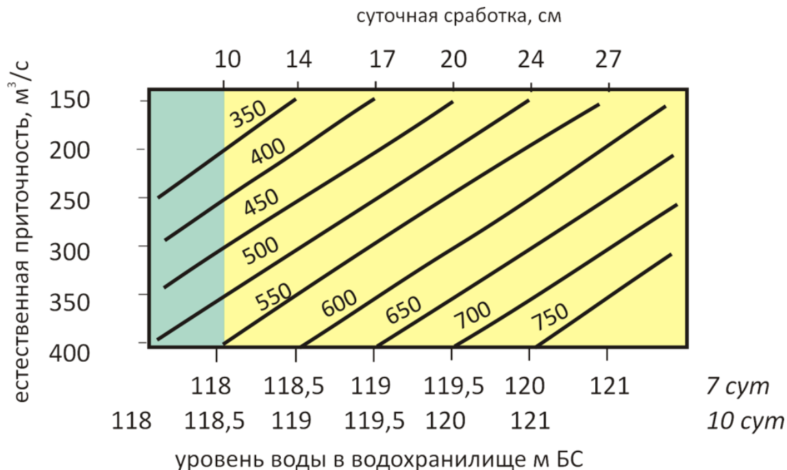
Рисунок 4. Номограмма достижимого максимального расхода воды (значения на линиях номограммы в м³/с) попусков с продолжительностью пика 7 и 10 суток в зависимости от естественного притока воды и допустимой суточной сработки уровня воды в водохранилище.
