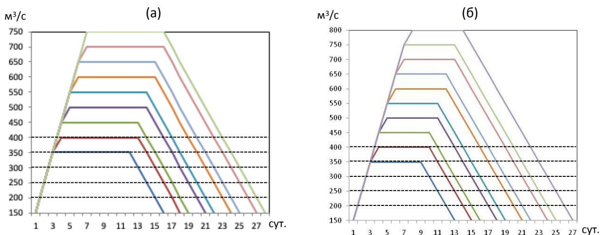
Рисунок 6. Гидрографы попусков различного объема с десятидневной (а) и семидневной (б) продолжительностью пика и суточным изменением расхода 100 м 3 /с на подъеме и 50 м 3 /с на спаде
